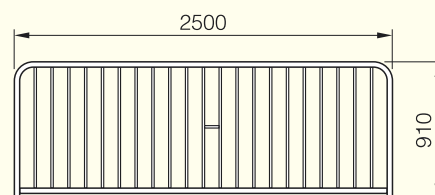
Barriärräcke Profil, vikt 18 kg
